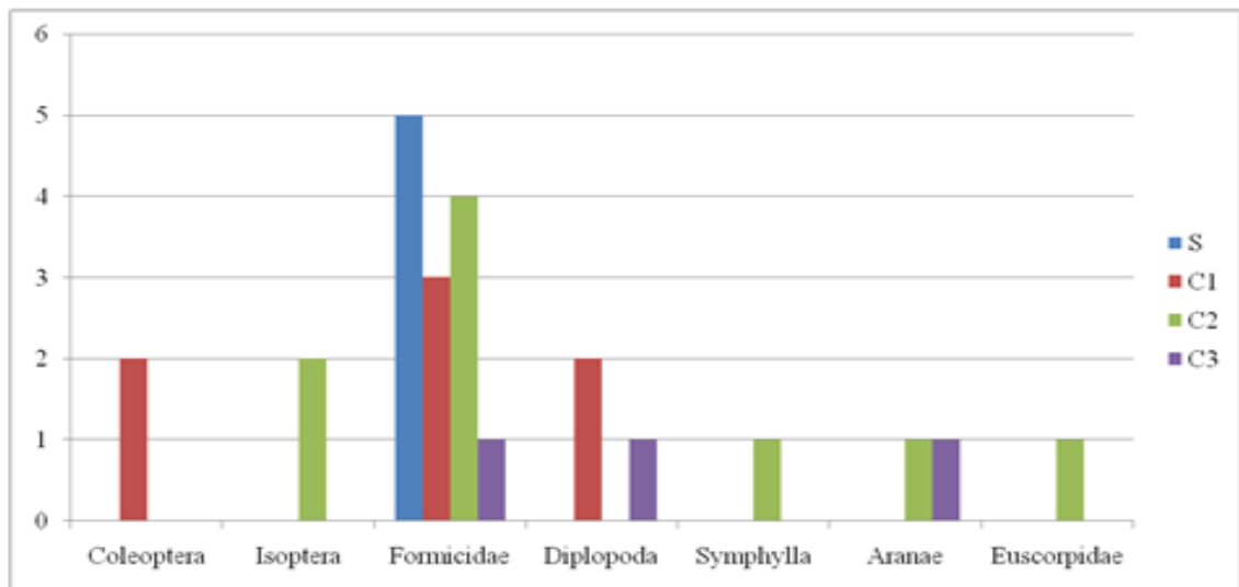
FIGURA 1 - Distribuição da macrofauna do solo nas diferentes camadas de solo, S: serrapilheira, C1: 0 – 10 cm, C2: 10 – 20 cm, C3: 20 – 30 cm, em área submetida a queimada no município de Sambaíba – MA, 2016.
