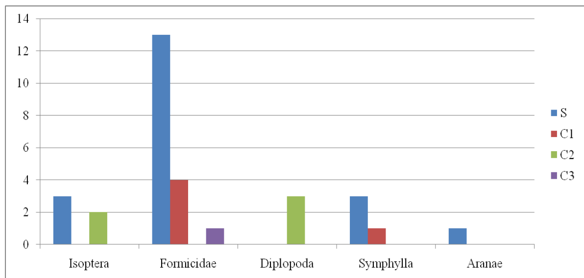
FIGURA 2 - Distribuição da macrofauna do solo nas diferentes camadas de solo, S: serrapilheira, C1: 0 – 10 cm, C2: 10 – 20 cm, C3: 20 – 30 cm, em área de pastagem Panicum maximum cv massai no município de Sambaíba – MA, 2016.
